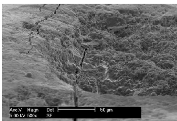
Figura 11 - Zona de grande erosão e fendas várias da superfície do esmalte duma amostra do grupo 3
