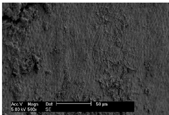
Figura 10 - Fenda na superfície do esmalte (visível no canto superior esquerdo da figura) duma amostra do grupo 2
