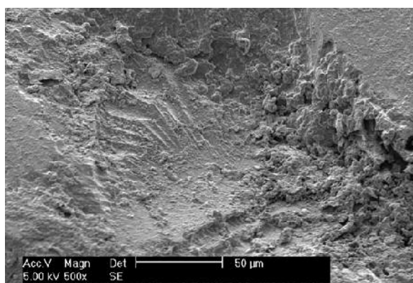
Figura 12 - Zona de grande erosão com aspecto de cratera da superfície do esmalte duma amostra do grupo 3
