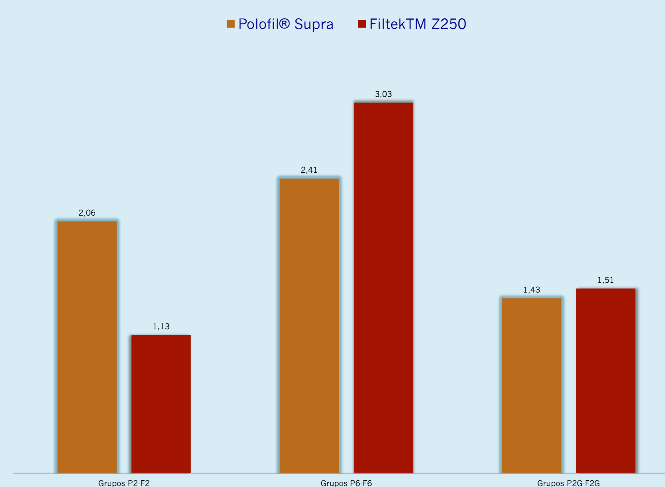
Figura 7 – Valores obtidos nas resinas Polofil Supra e Filtek Z250 . Todos os valores se encontraram entre 1,0 e 3,3 (intervalo de aceitabilidade).
