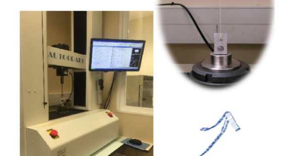
Figura 5 - Máquina de testes universais e respetivo teste à tração.
