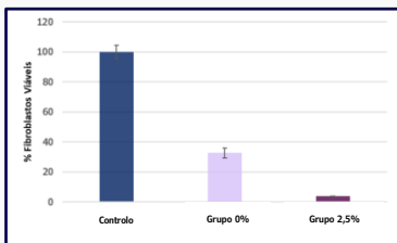
Ensaio de viabilidade por contato direto dos espécimes sobre a camada monocelular às 24h de cultura. (controlo vs experimental - p<0,01 )
