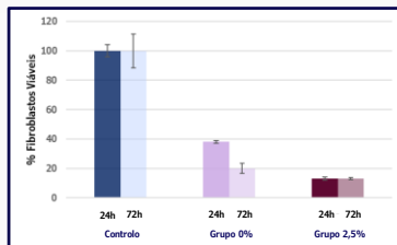
Resultados obtidos às 24h e às 72h de incubação no ensaio de proliferação celular sobre os espécimes. (grupo 0% - 24h vs 72h p<0,01 ; grupo 2,5% - 24h vs 72h p=0,02 )
